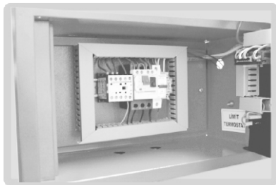
KUMANDA PANOSU İÇ GÖRÜNÜŞ
