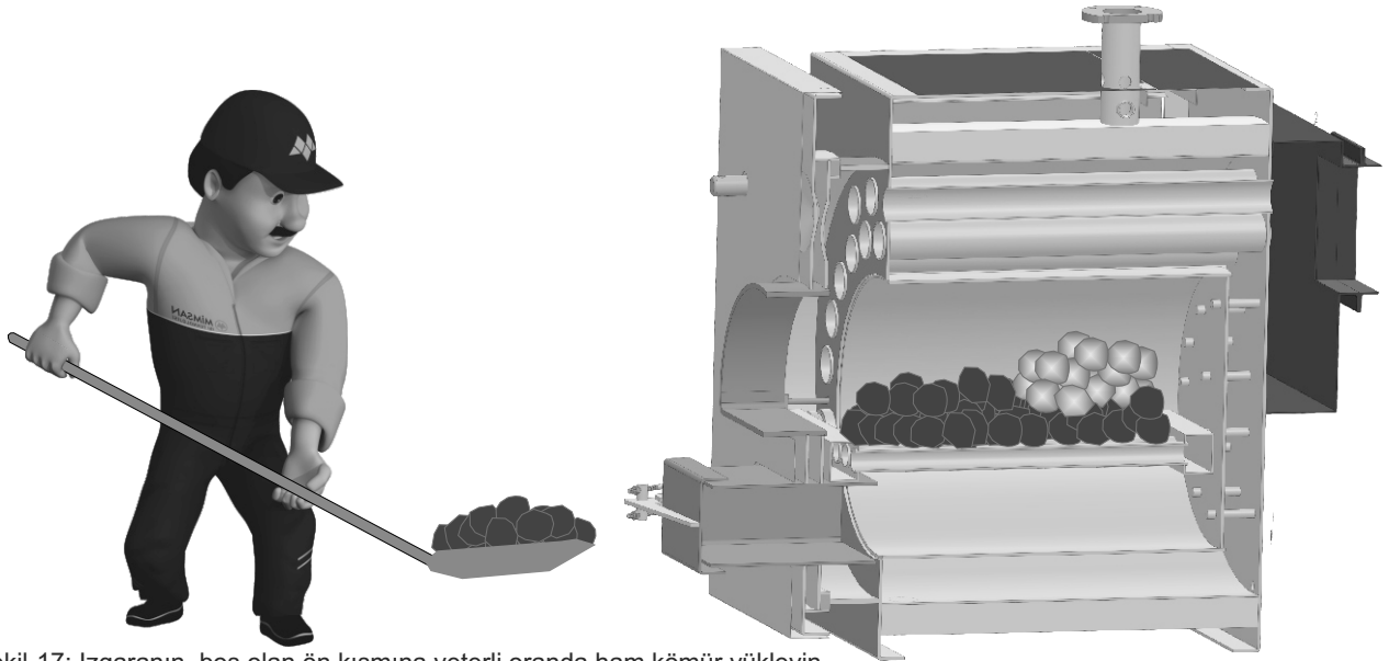
Şekil-17: Izgaranın, boş olan ön kısmına yeterli oranda ham kömür yükleyin.
